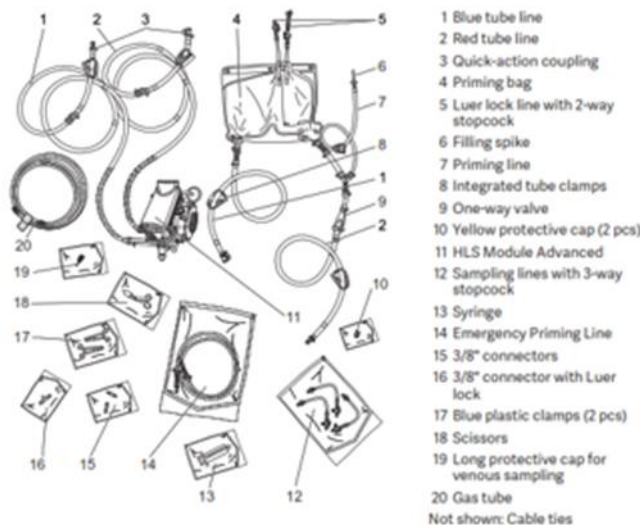
Figure 1 : Ligne de tubulure bleue (1), Emergency Priming Line (14)
